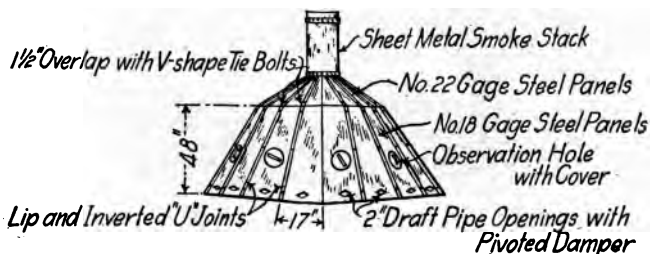
Fig. 14a. The Hubbard Stump Burner
